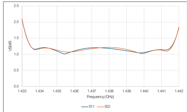
VSWR
